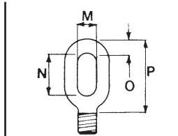
Swivel øje Swivel eye Cáncamo giratorio
